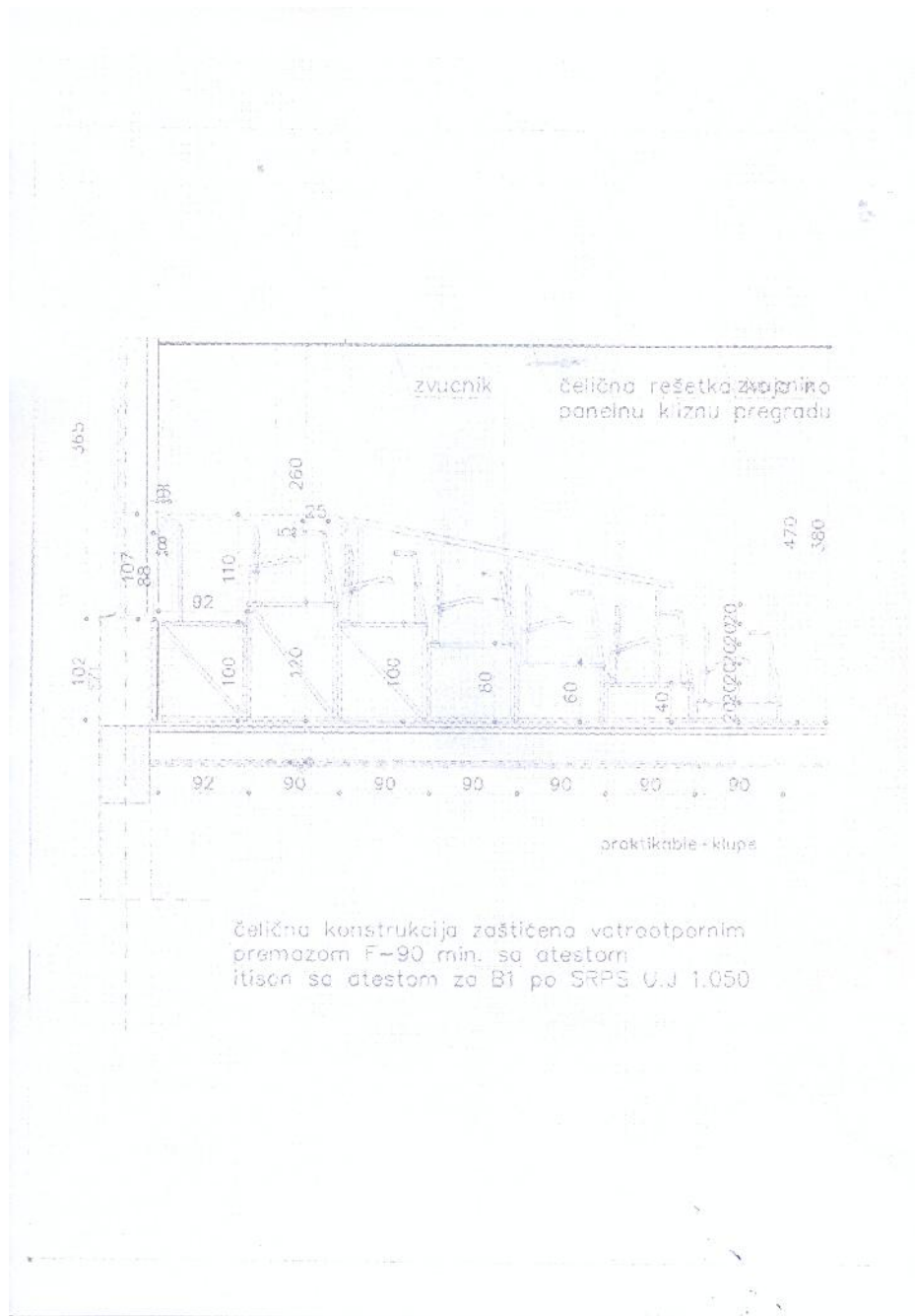
Конструкција подијума у амфитеатру
